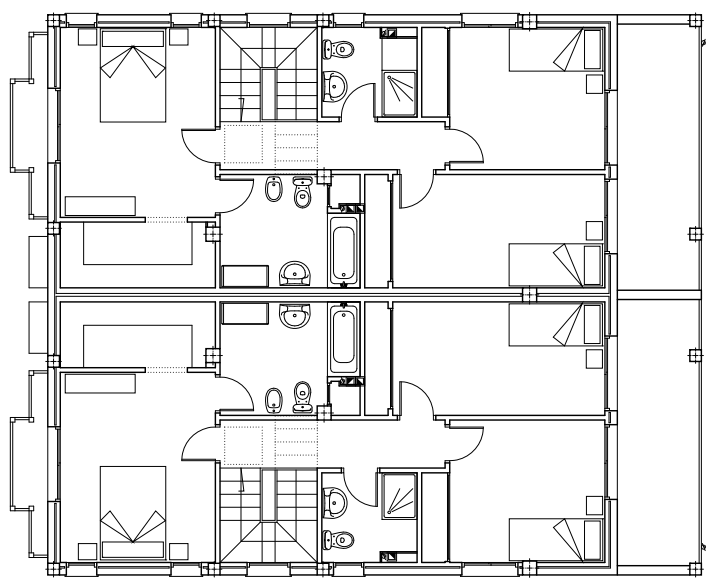
PLANTA PRIMERA
